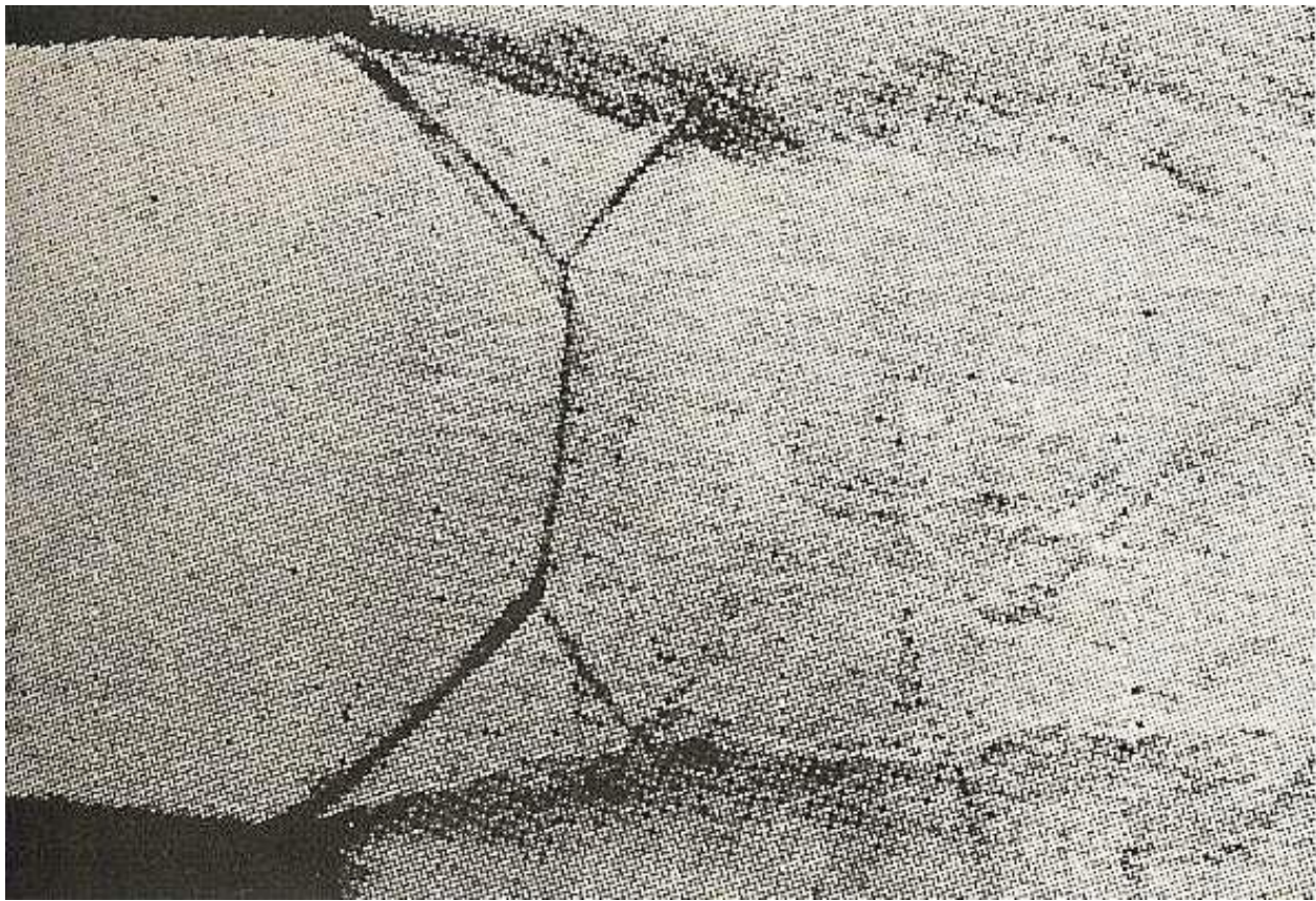
Foto Schlieren che mostra l’intersezione di onde d’urto a doppio \lambda all’uscita di un ugello
