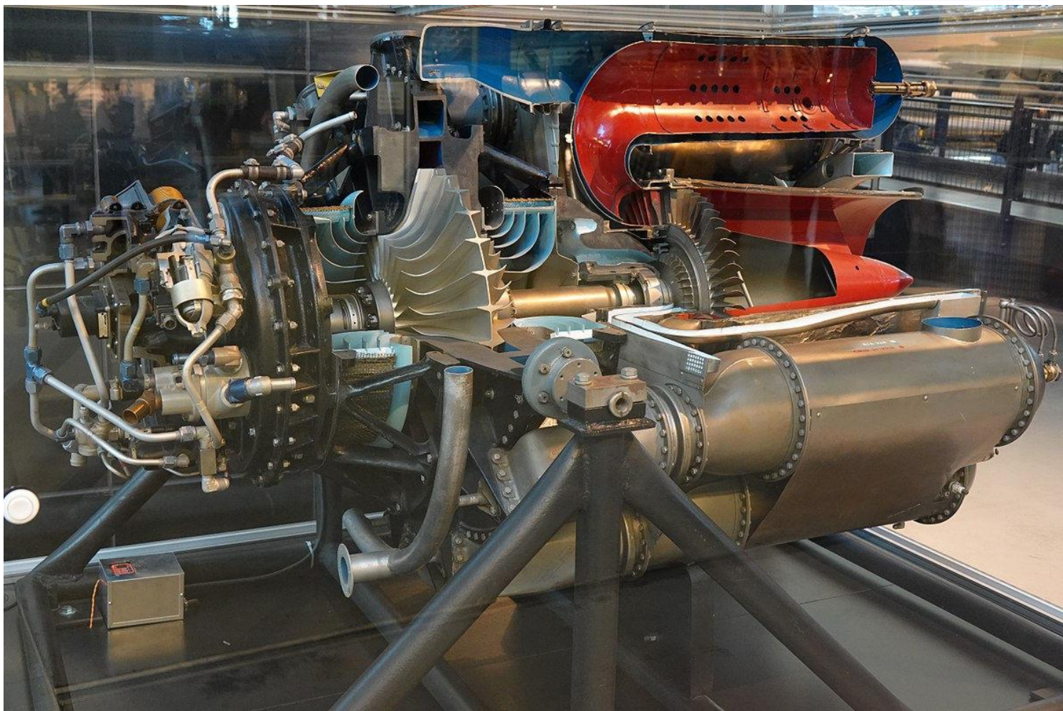
TurboJet
