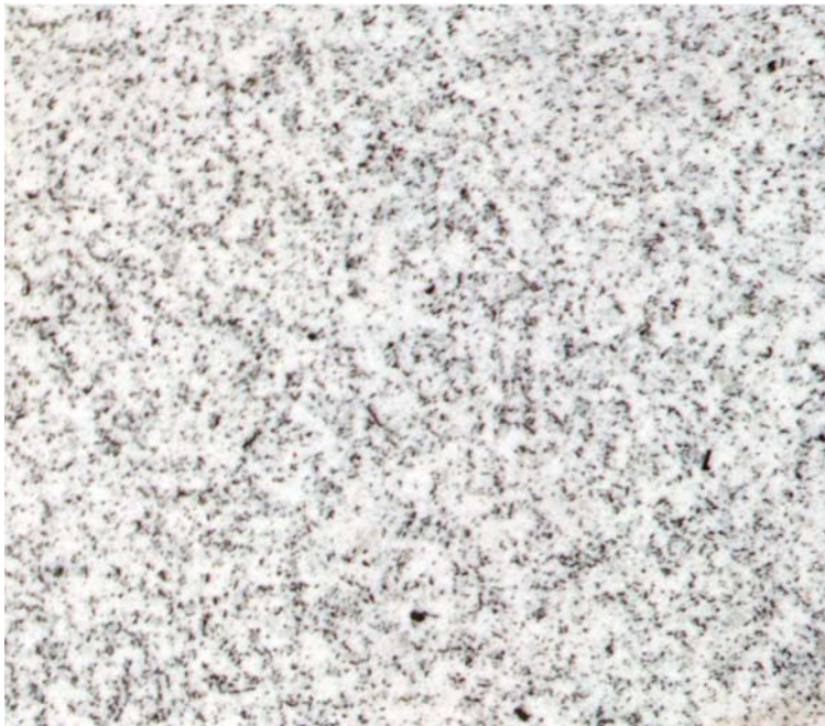
Aplite
