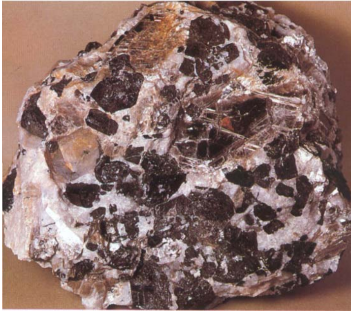
Pegmatite
