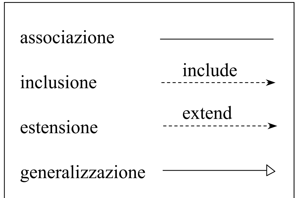
Relazioni nel diagramma degli use case
