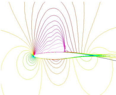
Iso-Mach contours.
