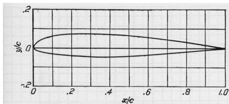
NACA 23012 airfoil
