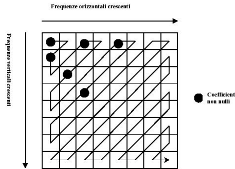
Figura 31: Scansione a zig-zag.
