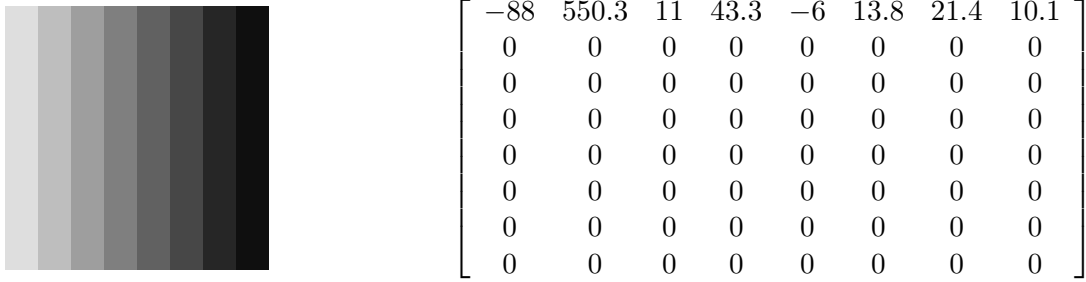
Figura 26: Blocco 8 \times 8 e relativi coefficienti DCT.
