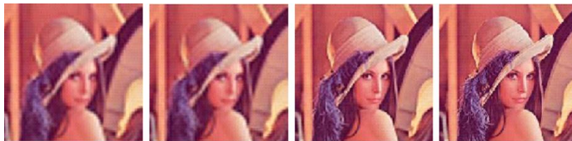
Figura 23: Codifica progressiva.
