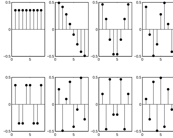
Figura 24: vettori riga della matrice \mathbf{C} per N = 8 .
