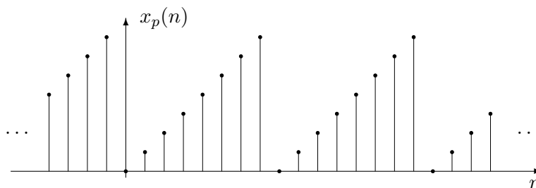
Figura 19: Estensione periodica.
