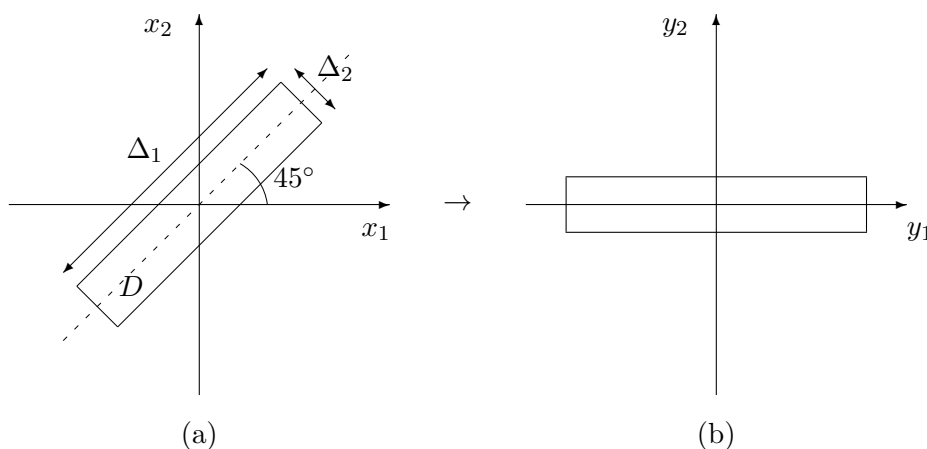
Figura 16: pdf congiunta, componenti correlate (a) componenti incorrelate (b)
