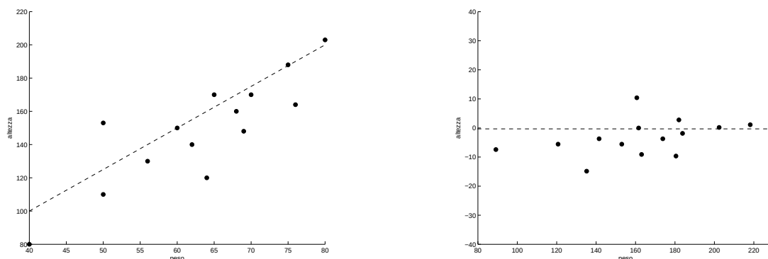
Figura 15: Rappresentazione grafica della coppia peso e altezza.
