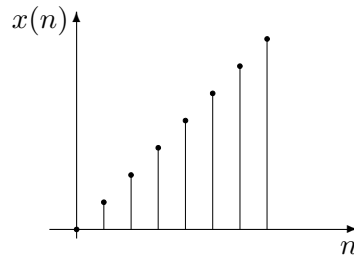
Figura 18: Segnale da trasformare.
