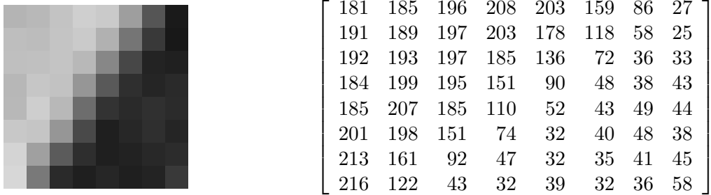
Figura 35: Blocco ricostruito.
