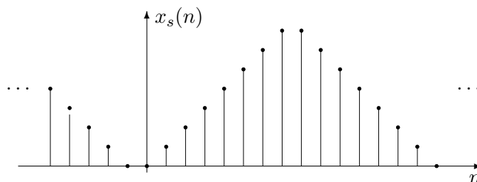
Figura 20: Estensione simmetrica.
